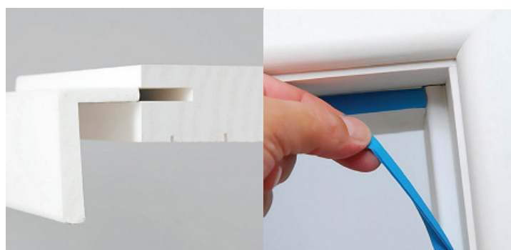
Figura 2: Batente para receber guarnição regulável.
